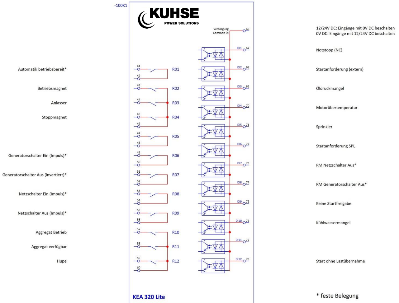
Abb. 7: Anschlussplan 2 der KEA 320 RP LITE / KEA 320 LITE
