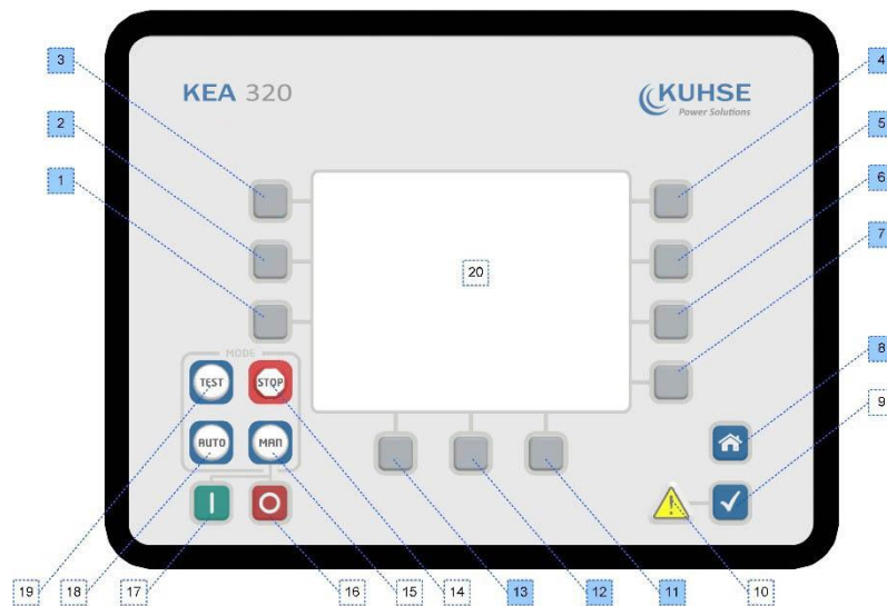
Abb. 11: Bedienfeld und Display
