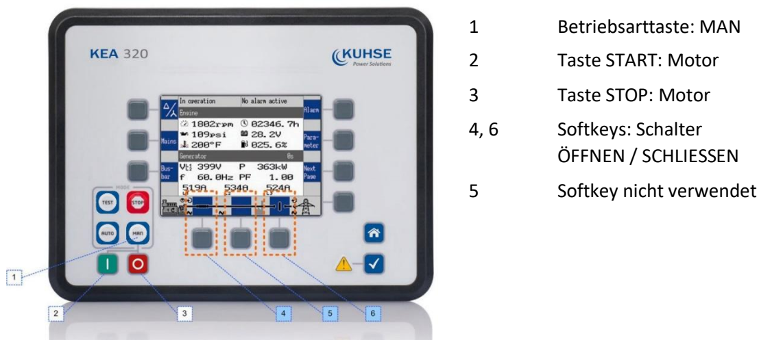
Abb. 10: KEA 3X0 MAN-Tasten
