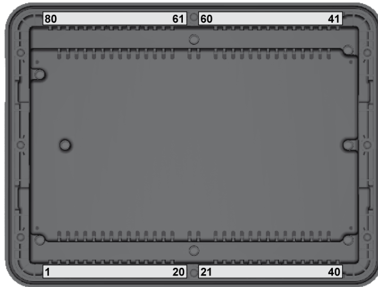
Abb. 4: Klemmen des KEA 320 LITE (Kunststoffgehäuse)
