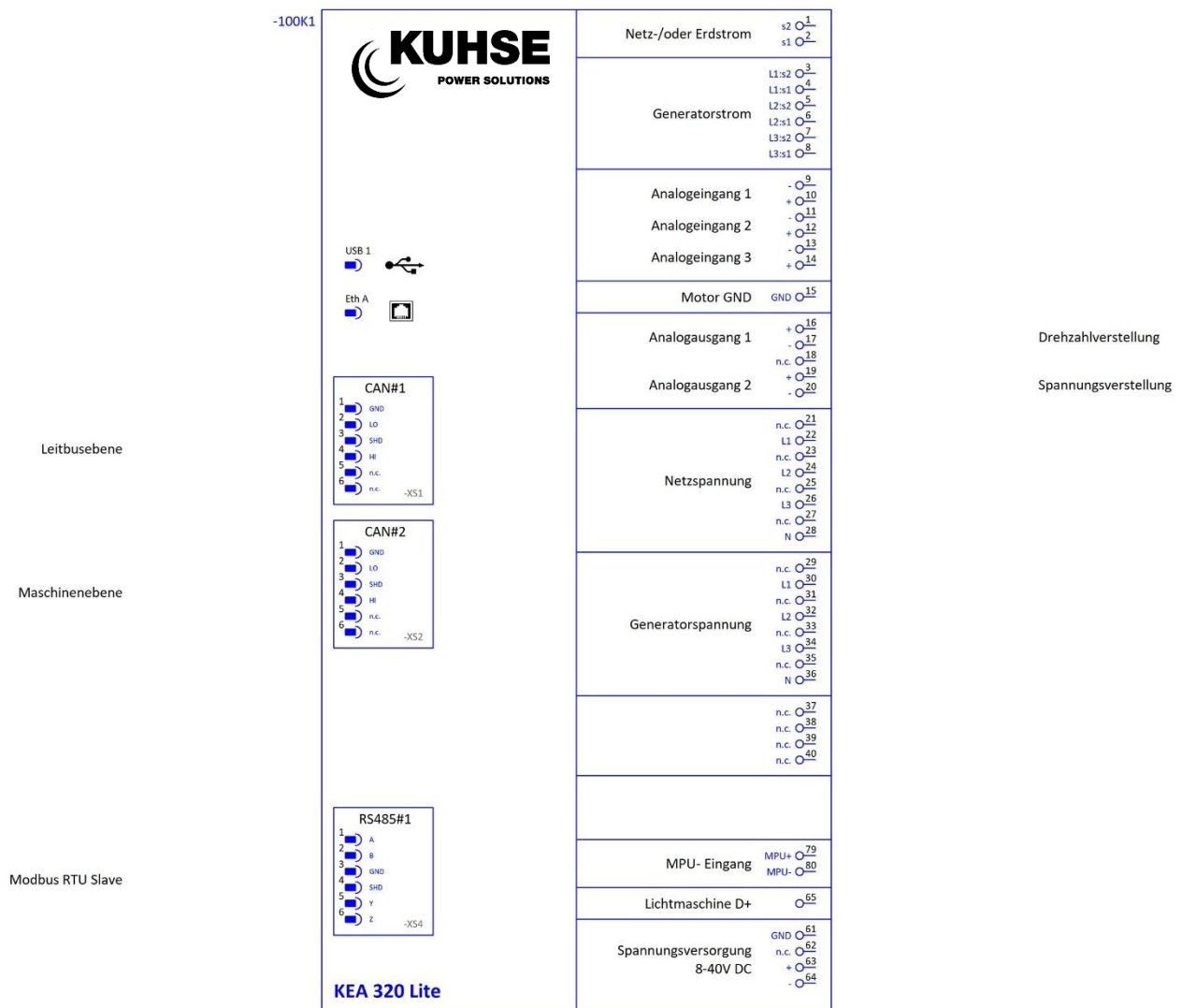
Abb. 6: Anschlussplan 1 der KEA 320 RP LITE / KEA 320 LITE
